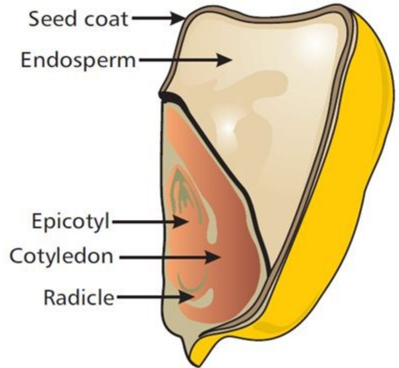
Monocotyledon
